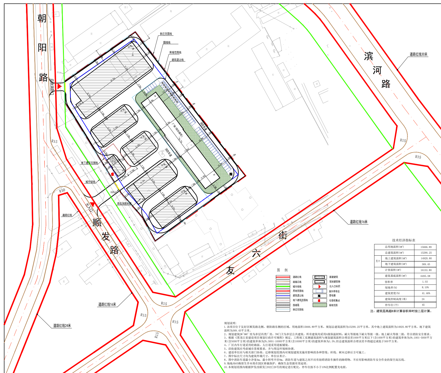
修详总平面图
