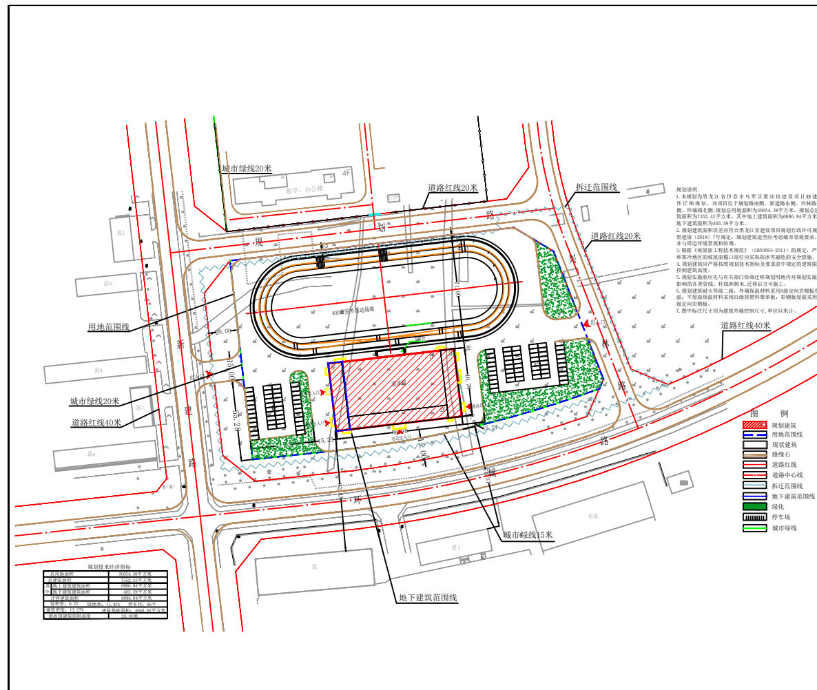
总平面图
