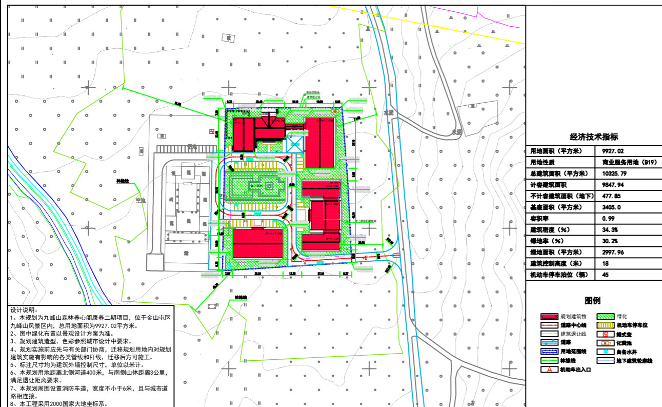
—总平面规划图
